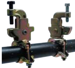
H 鋼クランプ (直交 / 自在) [I Beam Steel Clamp (90°fixed / Swivel)] 価格 ¥300
