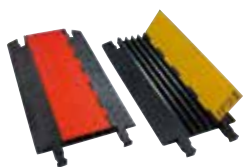
ケーブルマット [Cable Protector Ramp] ・ 5 レーンタイプ 9.8kg W:500×H:50×1000mm ・ 4 レーンタイプ 9.3kg W:455×H:50×1000mm 価格 ¥2,000
